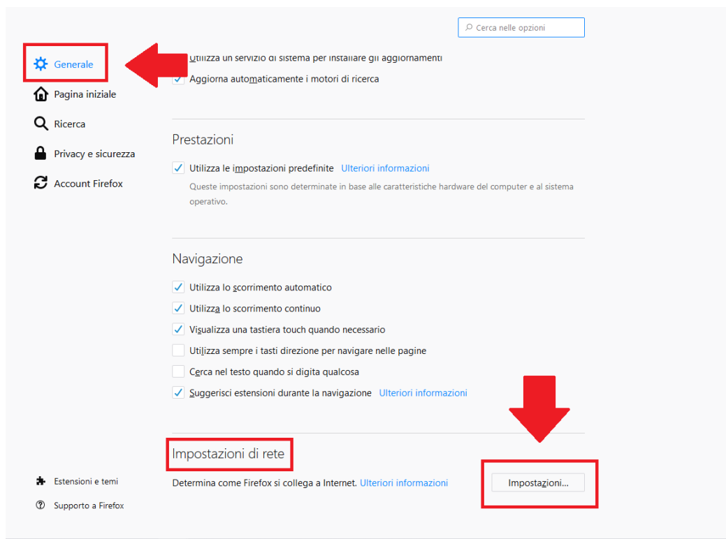
Figura 2 – Generale - Impostazioni.
