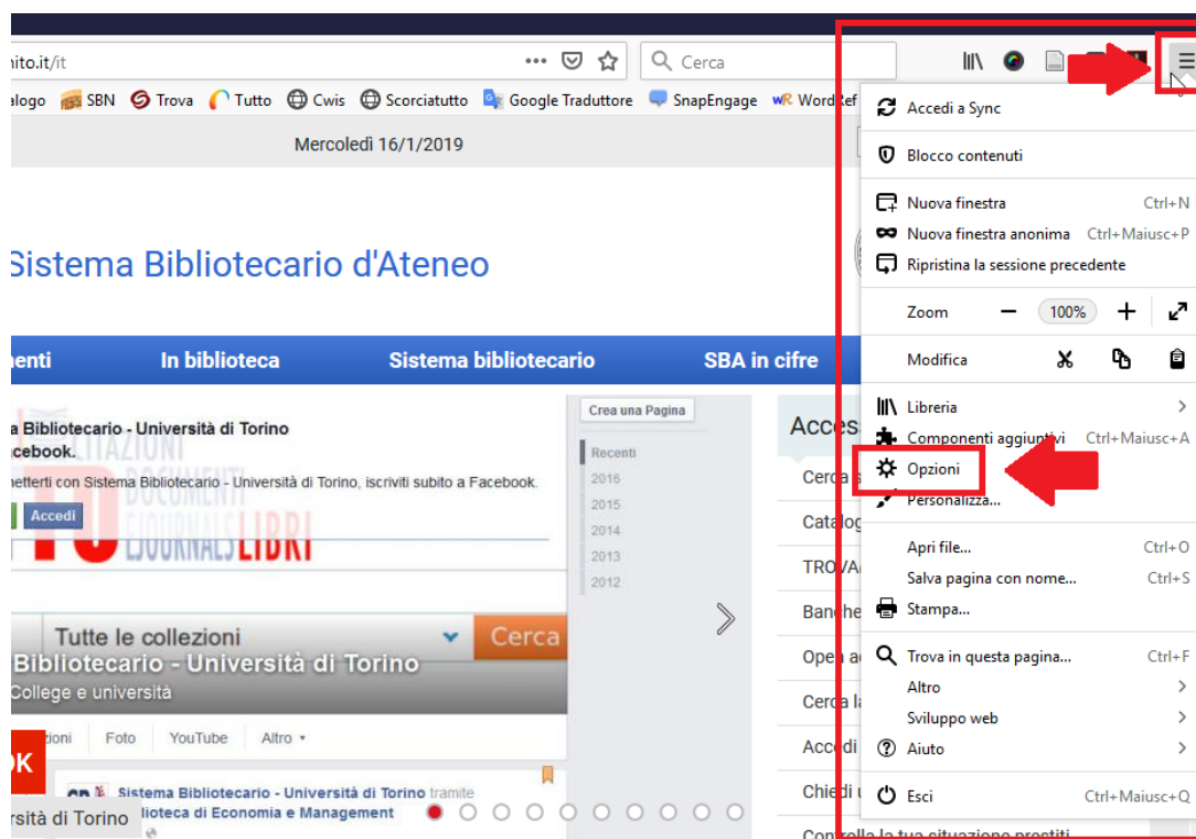
Figura 1 – Opzioni.
